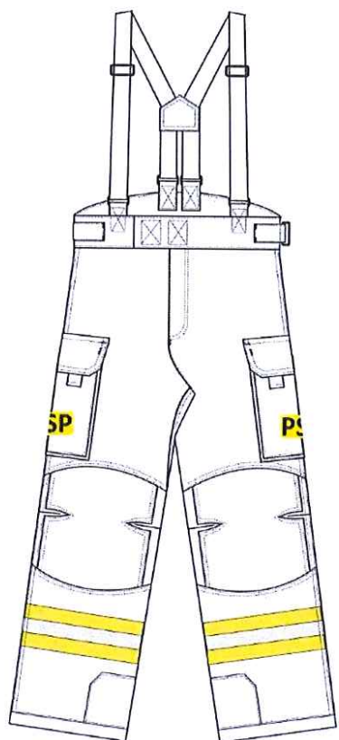
Rys. 3 Widok spodni z przodu
